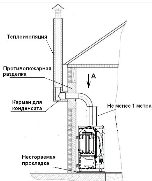
Схема подключения к дымоходу
