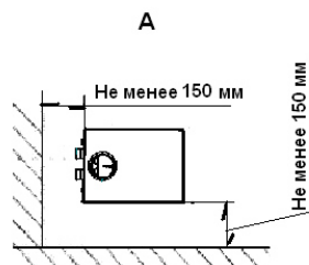
Схема установки котлов
