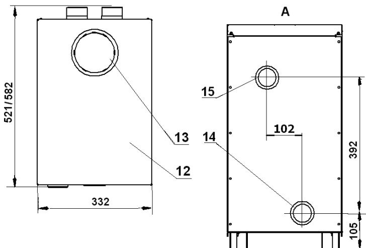
Рис.2 Котлы КС-Г-16S-Э/20S-Э/16Т-Э/20Т-Э Остальное см. рис. 1
